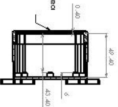
A-A (1 : 1.5)
